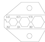
Die profile
