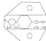
Die profile
