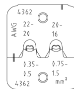
Die profile
